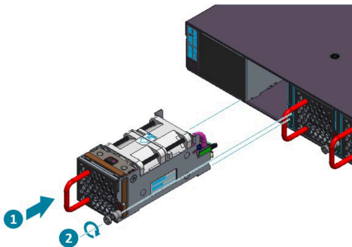
Figure 2.9. Inserting the fan module
