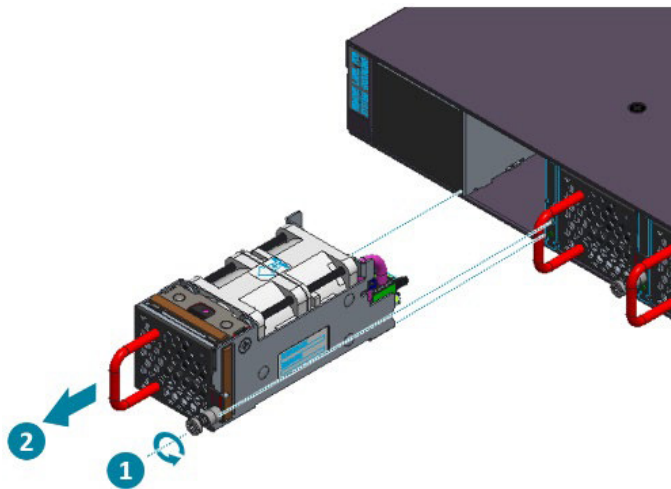
Figure 2.8. Removing the fan module
