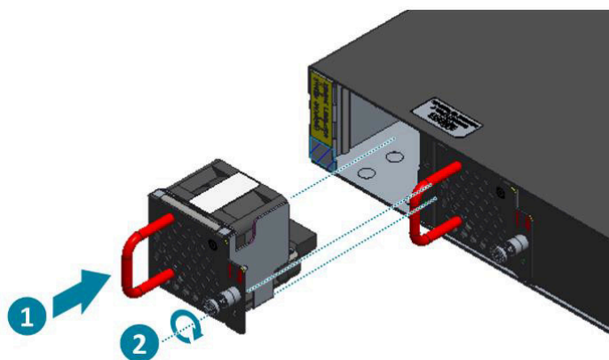
Figure 2.8. Inserting the fan module
