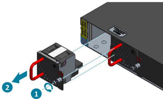
Figure 2.7. Removing the fan module
